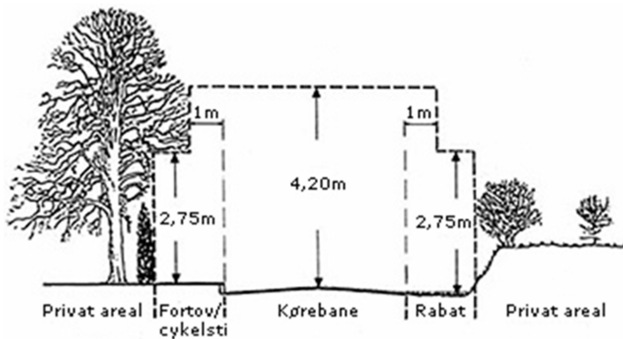
Illustration af afstande til fortov og kørebane samt højder for hække og træer.
