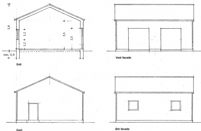
Figur 2 Facadetegning
