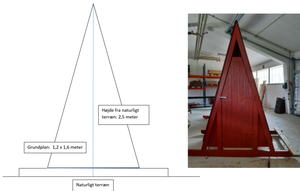
Figur 2 Facadetegning
