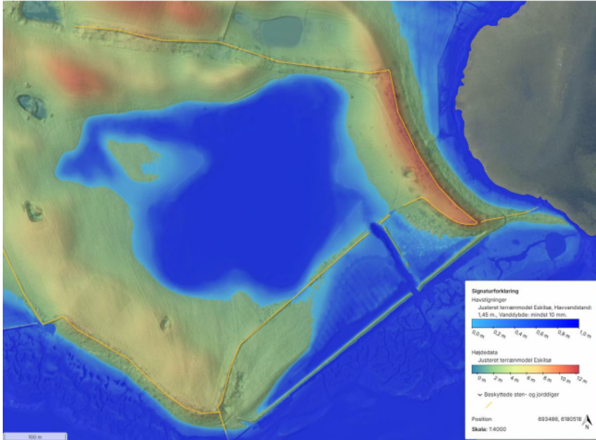
Figur 2 Returperiode der forekommer 1 gang hvert 2. år svarende til en vandstand på 1,45 m inkl. det beskyttede sten- og jorddige (gul streg), som vil blive delvist oversvømmet ved denne hændelse.
