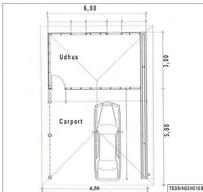
Eksempel på plantegning
