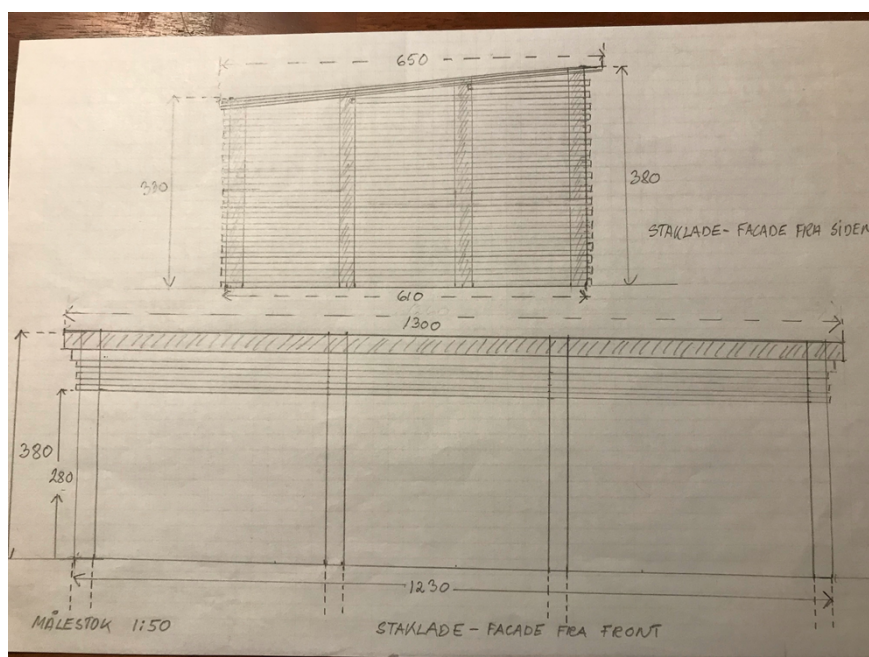
Figur 3 facadetegning
