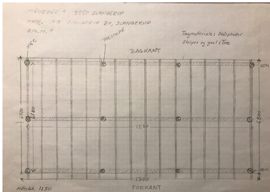
Figur 2 grundplan
