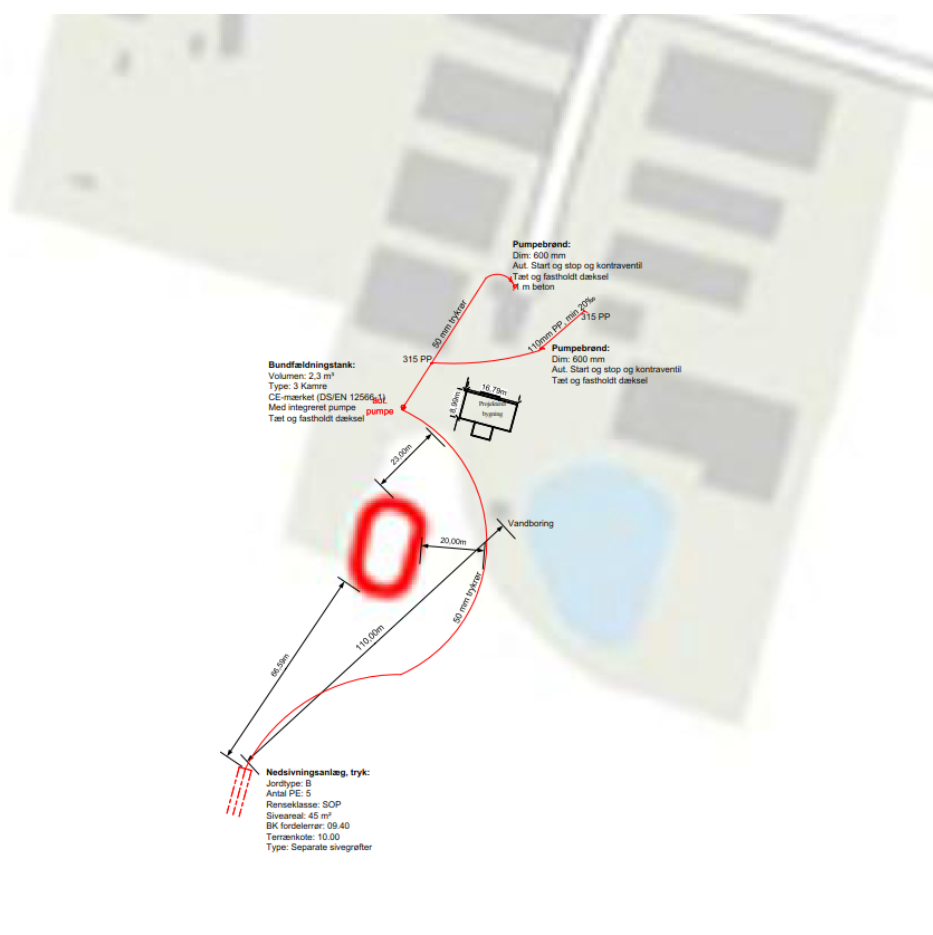
Figur 1 Rød cirkel viser det beskyttede fortidsminde, den røde linje er et 50 mm trykrør, der løber fra pumpebrønden via bundfældningstanken til nedsivningsanlægget. Der holdes en afstand mellem trykrør og fortidsmindet på minimum 20 meter og 66 meter til nedsivningsanlægget.
