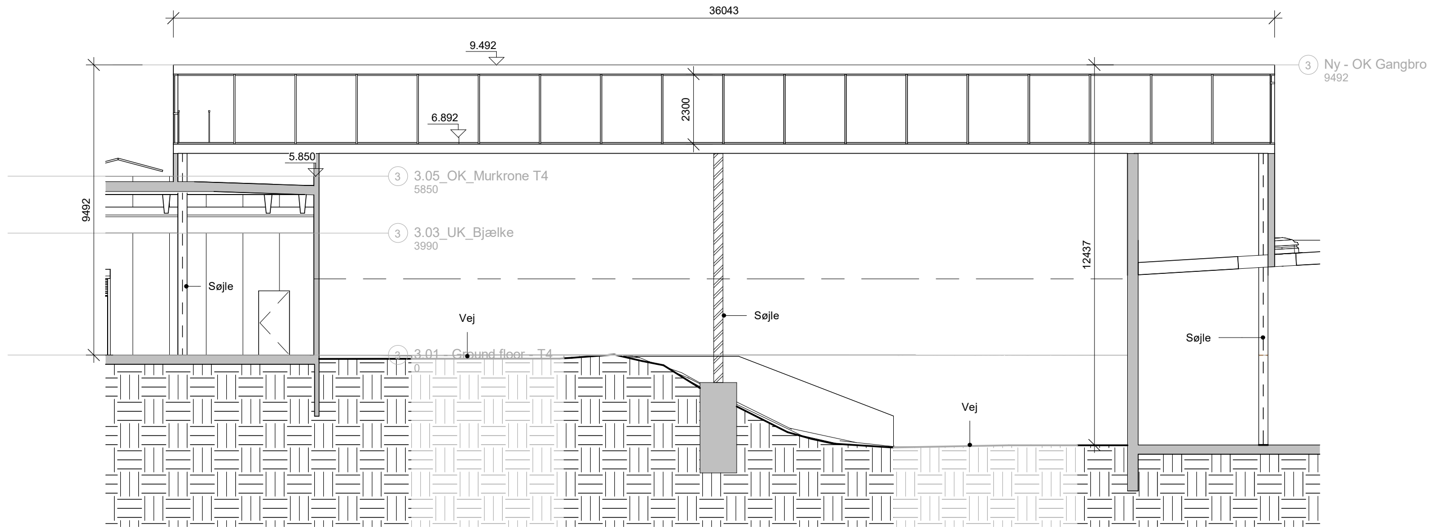
Snit A-A - Ny gangbro 1 : 125
