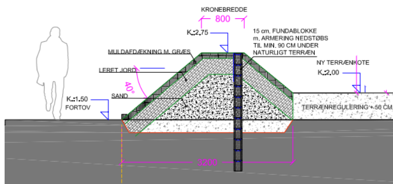
Figur 2: Principsnit af kystbeskyttelsesanlæg, med højvandsmur, samt for- og bagdige i jord. Skal opdateres med T-sikringsløsning
